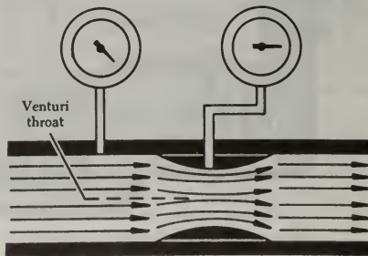
FIGURE 3-4. Simple venturi.
